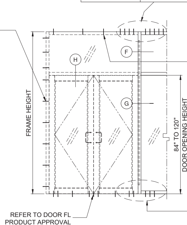
DOUBLE DOOR JAMB ANCHORS
