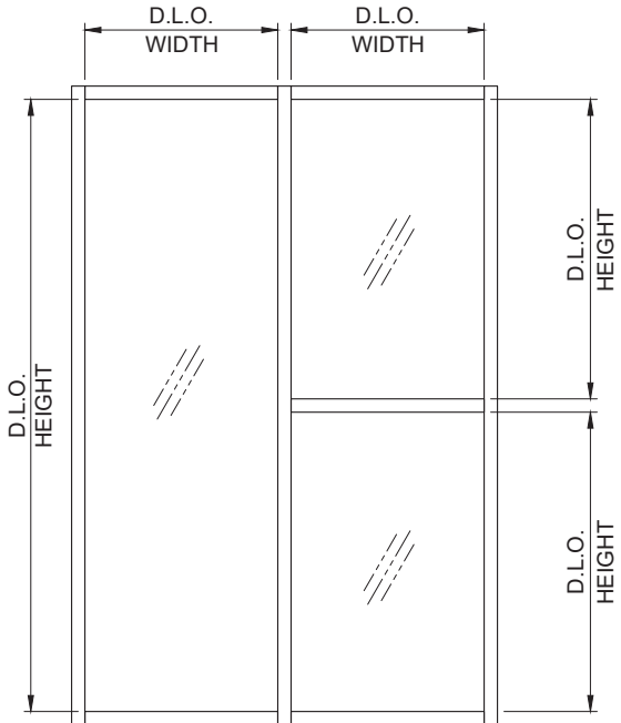
ELEVATION 1
