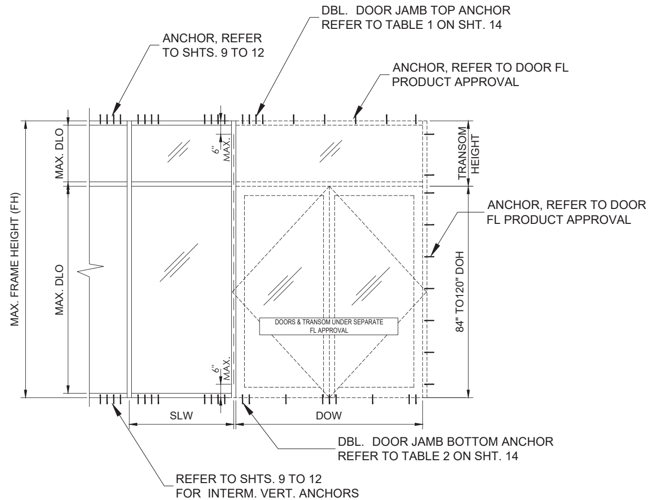
ELEVATION 4
